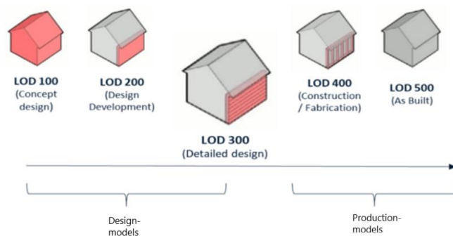
Bilde 1: Detaljeringsnivåer
